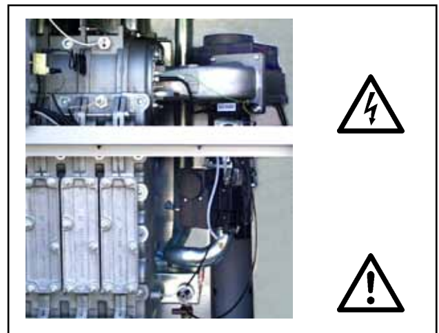
Bild: Zündtrafo, Hochspannungs-Zünder, Brennkammer Gefahr durch elektrische Spannung, Gefahr von Verbrennung durch heiße Bauteile
